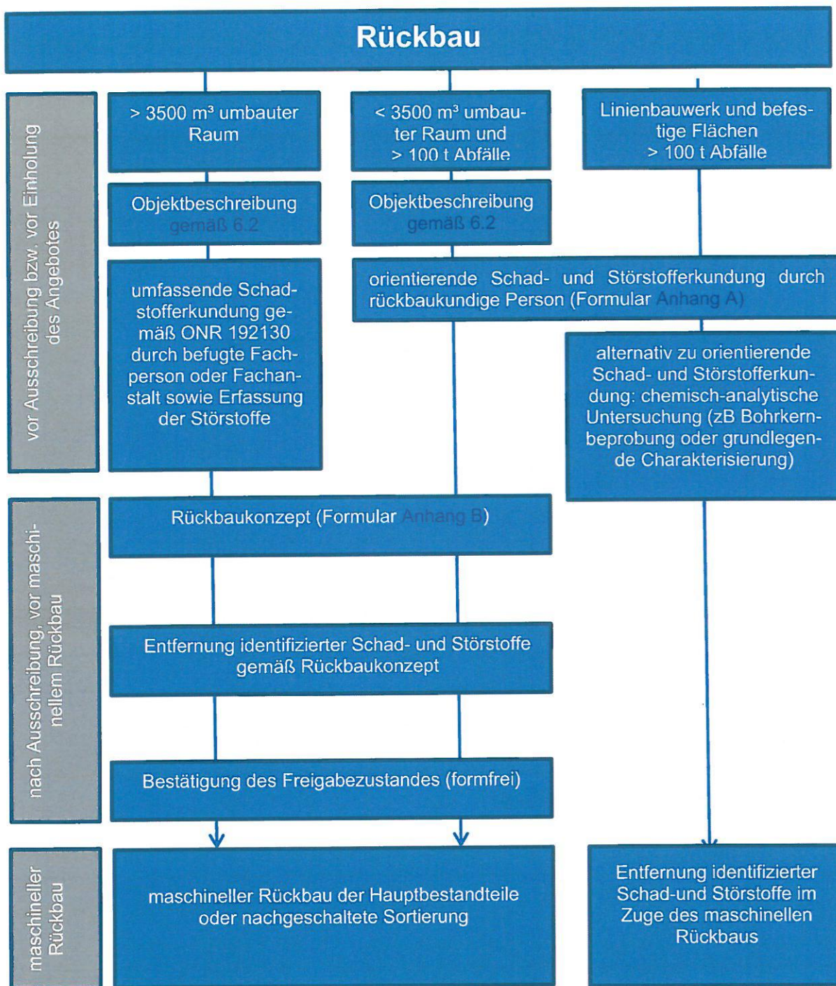
Bild C.1 — Rückbau
